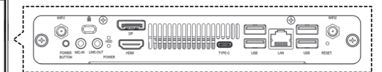
Optional OPS VPC35 / VPCF5 / VPC37 / VPC-A31
